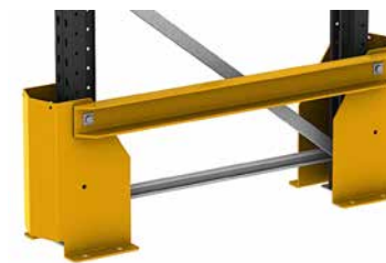
Volledige jukbeschermer PBS RKN/U
